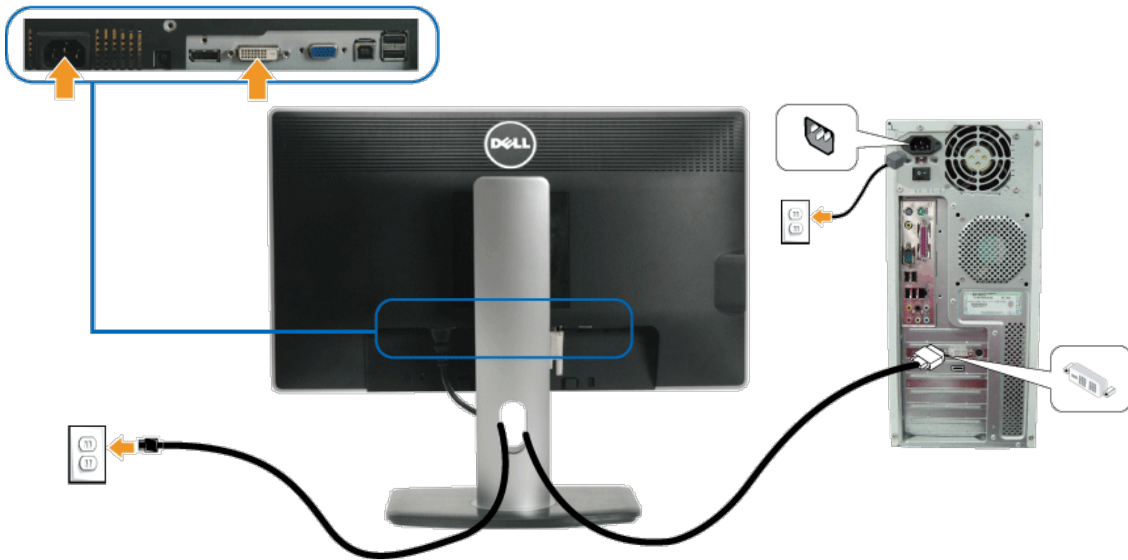
Подключение синего кабеля (VGA)
