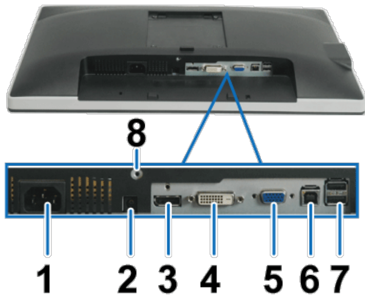
Вид снизу
